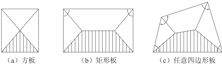
图 10.3.8 荷载分布图
