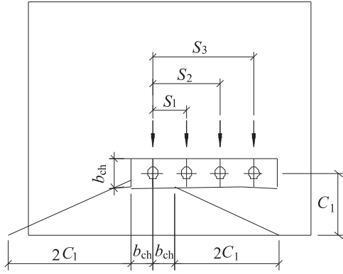
图 B. 0. 2—7 锚筋间距
